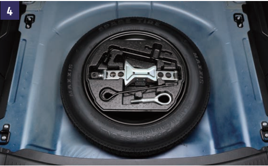
4 | Sada rezervního kola Pro řádnou montáž jsou potřeba všechny následující položky: 4-1, 2 a 3. 4-1 | Sada rezervního kola WVTA 48V Obsahuje pneumatiku, ventil, kolo, držák, informační leták, schránku s nářadím a zvedák. Objednací číslo 9929P-63T02-000 D E F H I 4-2 | Rukojeť zvedáku Objednací číslo 09827-00004-000 4-3 | Klíč na kola Objednací číslo 89921-83E00-000
